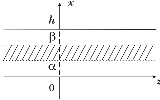
Рис. 1. Диэлектрическая пластина в плоском волноводе
