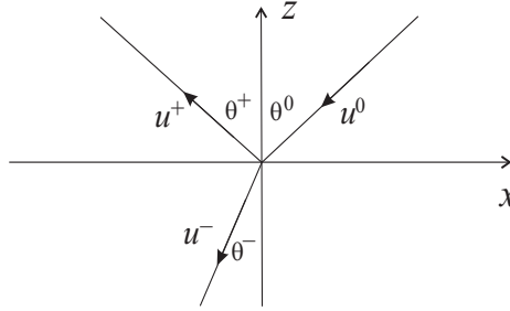
Рис. 2.1. Отражение и преломление плоской волны
