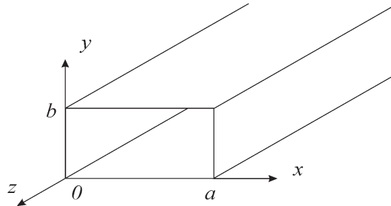
Рис. 3.2. Прямоугольный волновод
