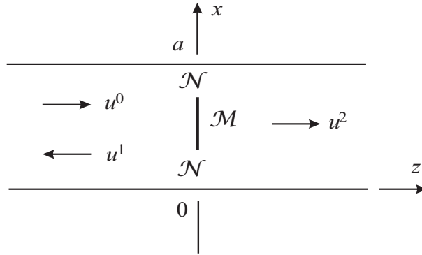
Рис. 4.1. Поперечная перегородка в плоском волноводе
