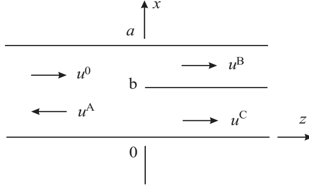
Рис. 4.2. Разветвление плоского волновода
