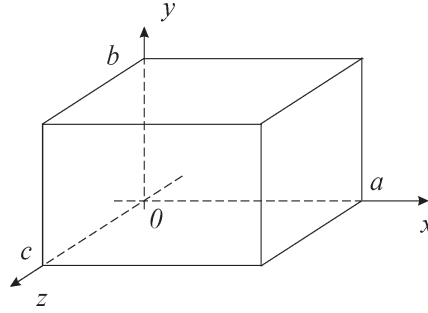
Рис. 3.3. Прямоугольный резонатор
